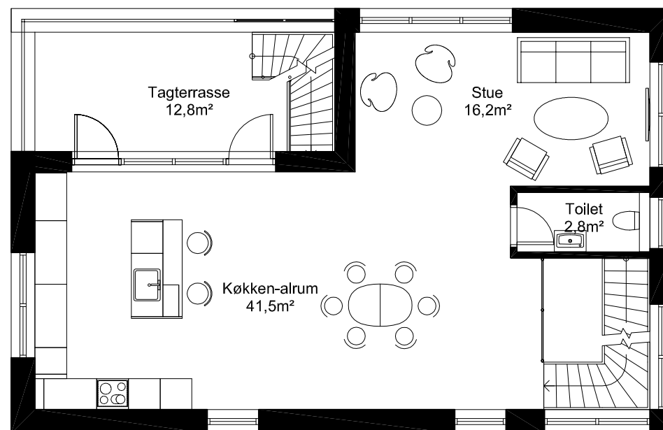
1. SALSPLAN 1:100
