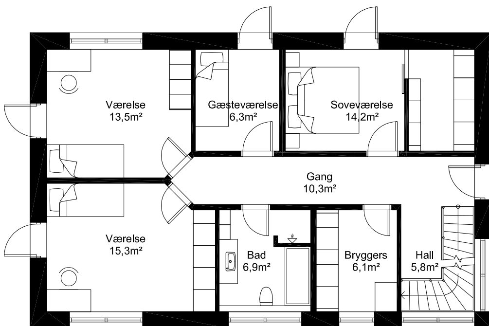
STUEPLAN 1:100
